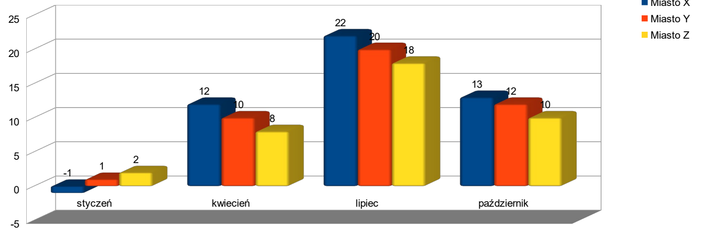
Temperatura powietrza w wybranych miastach Polski
