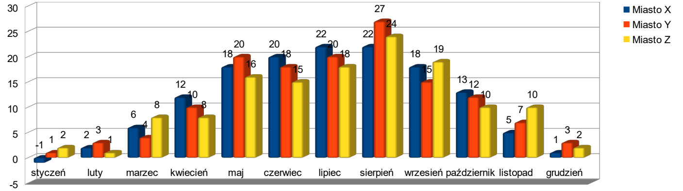
Temperatura powietrza w wybranych miastach Polski
